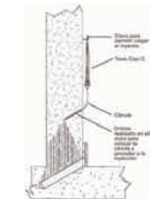
Esquema en sección del muro con la colocación del sistema de inyecciones
