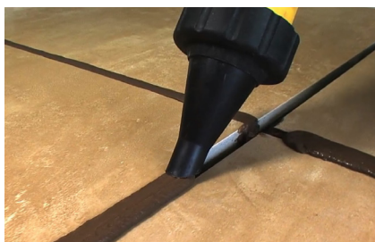
Jointoiement de brique et carreaux
