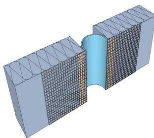
Teais Junta Systèm ITE
